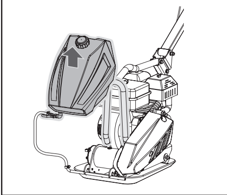
Rüttelplatte mit optionalem Wassersprühsystem
